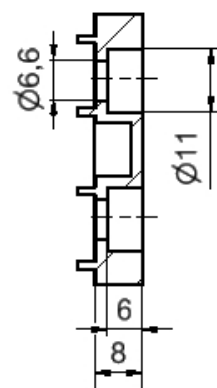
B-B ( 1 : 1 )
