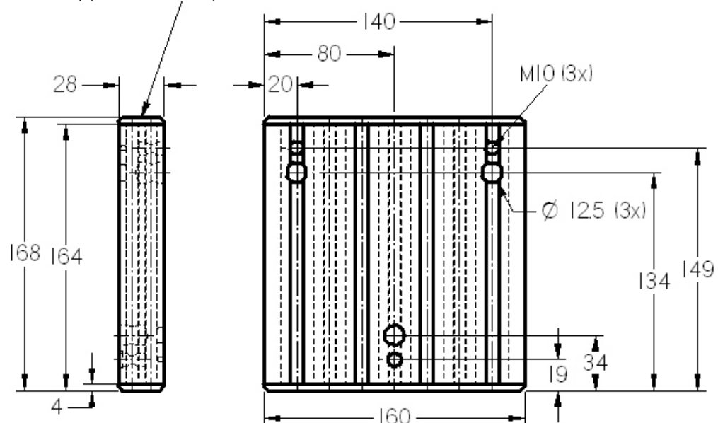
Abdeckkappe für Bodenplatte 160x160 (2x)
